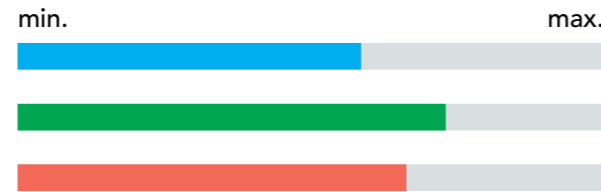
CÉRAMIQUE MARTENSITIQUE
